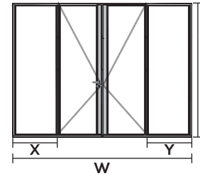
G. DOUBLE DOOR STANDARD + FIXED
