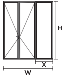
D. DOUBLE DOOR MINIMAL + FIXED
